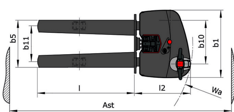
Stacky 10 S16 - Tekening met afmetingen
