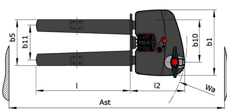
Stacky 10 D28 - Tekening met afmetingen
